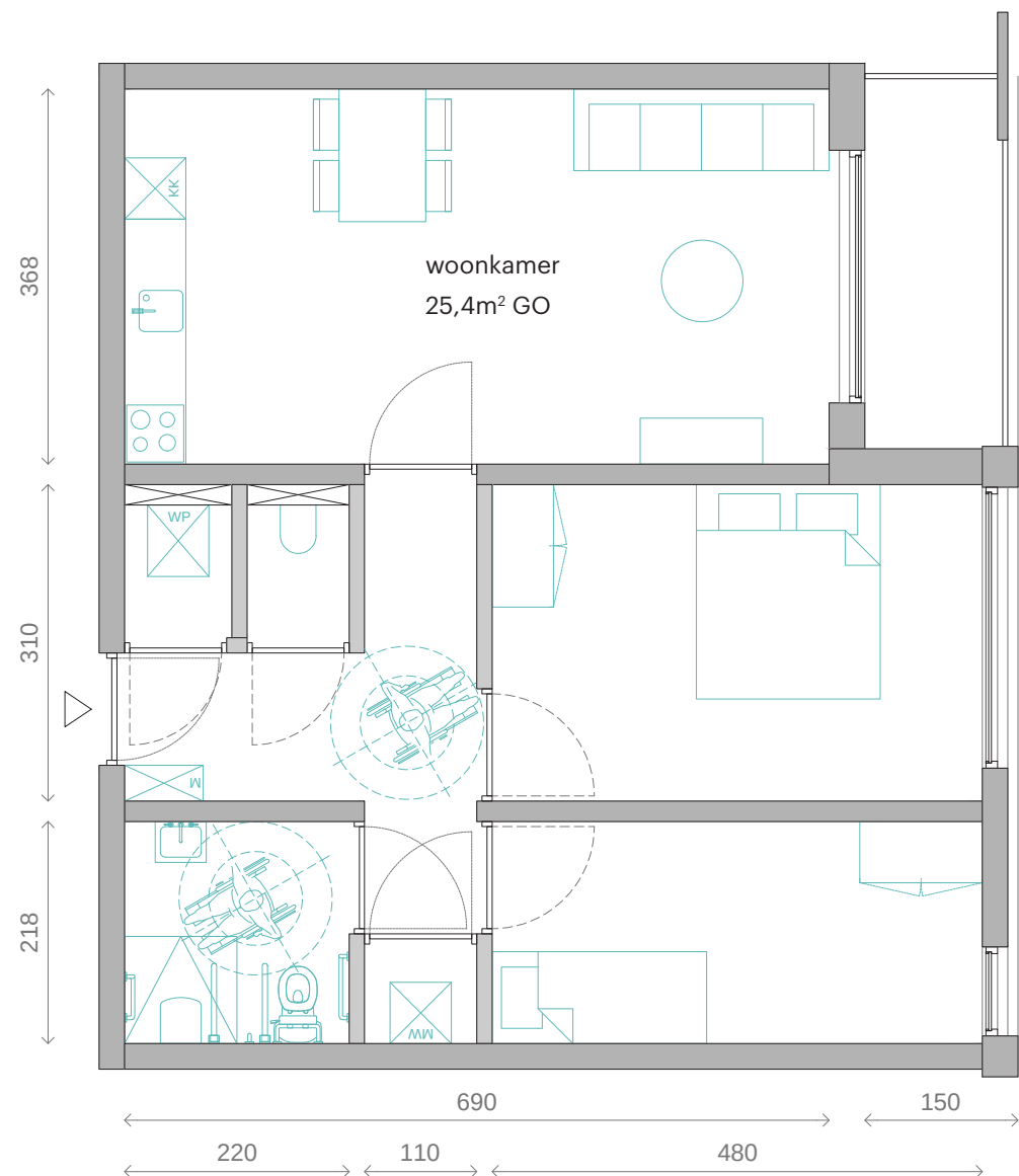
TYPE D PMC 7 LLB appartement, 2 slaapkamers, 70m²
