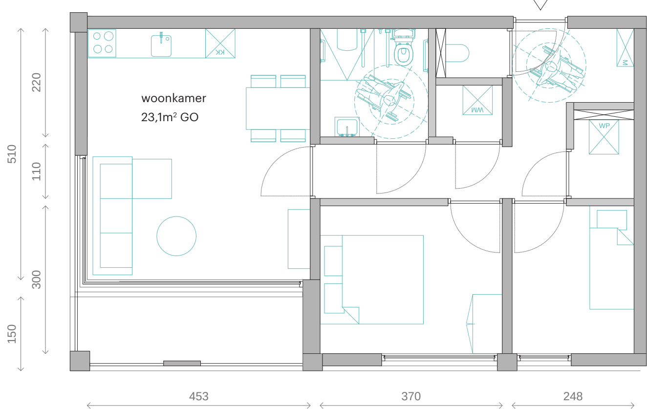
TYPE A PMC 7 LLB appartement, 2 slaapkamers, 68m²
