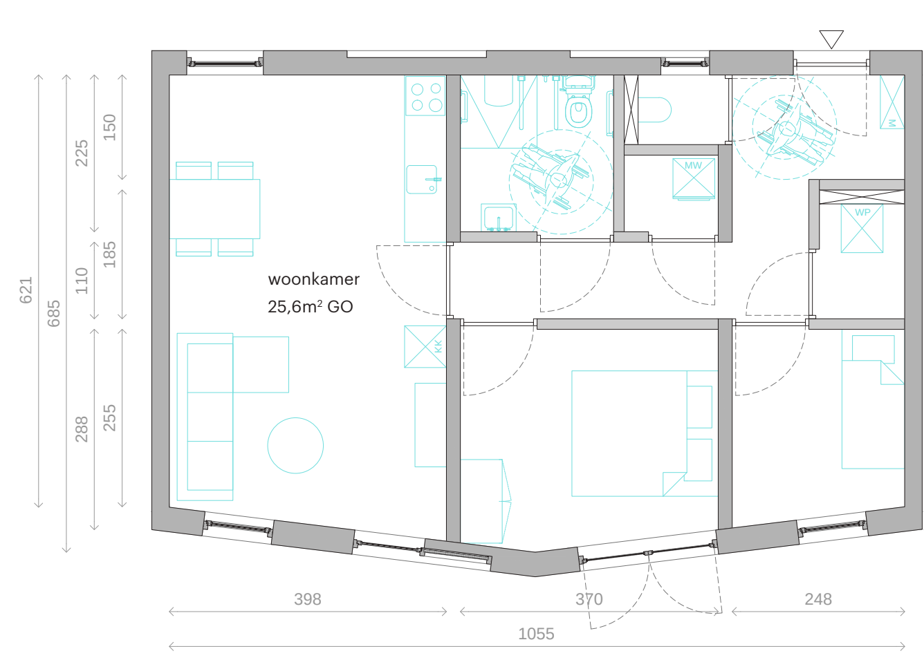
BEGANE GROND EN EERSTE VERDIEPING
