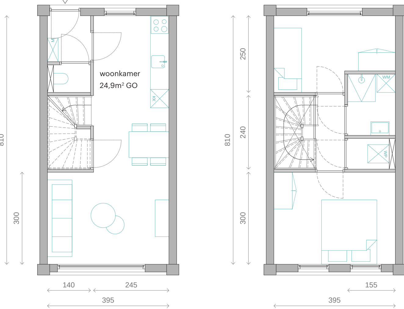
TYPE E PMC 2 kleine eengezinswoning, 2 slaapkamers, 64m²
